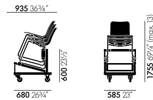
HAL Sledge, Schlitten-Stahlrohruntergestell, stapelbar, mit Reihenverbindung
